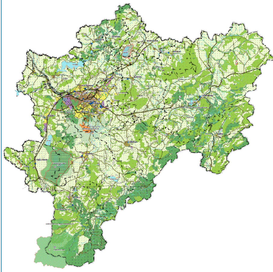
Kayseri İl Bütünü 1/50.000 Ölçekli Çevre Düzeni Planı
