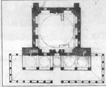
Kayseri Kurşunlu Cami Planı
