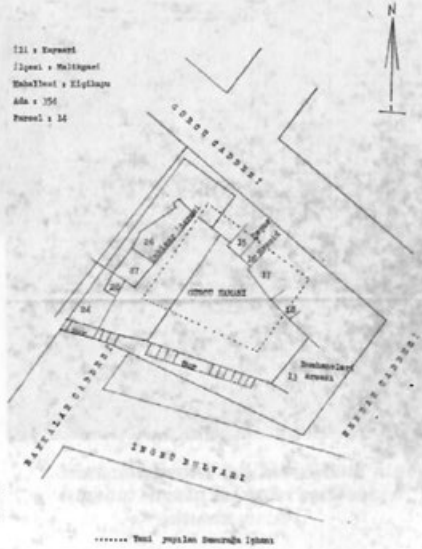
Gürcü Osman Paşa Hamamı Yeri Eski Durumu
