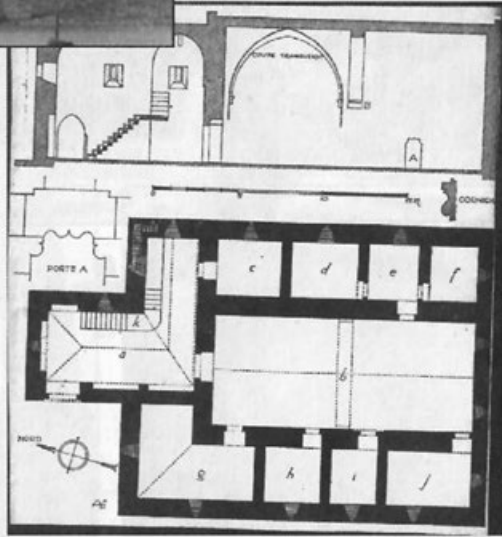
Haydar Bey Köşkü Planı (Gabriel'den)
